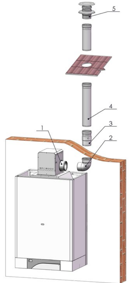
Дымоудаление 1x 100 выхлоп (вертик.)
